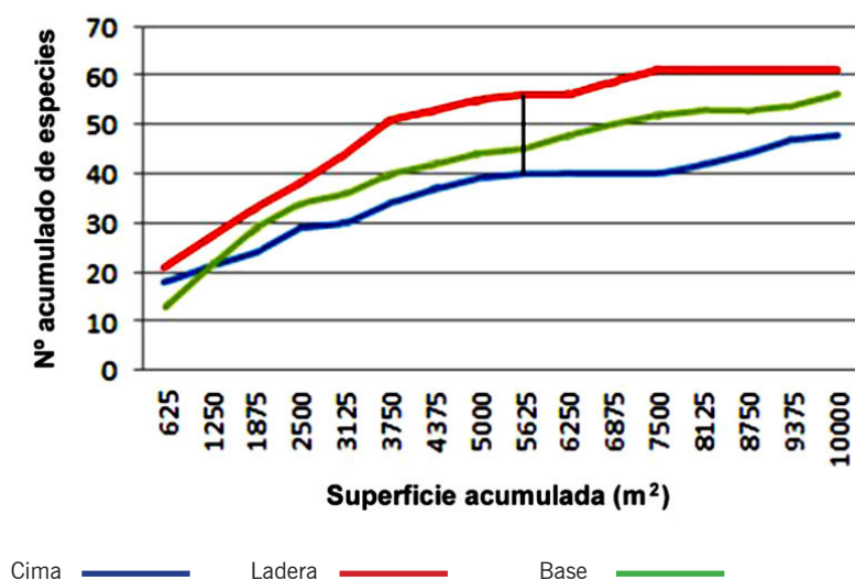
Figura 2. Curvas de especie-área que relacionan el número acumulado de especies (DAP \geq 10 cm) por unidad de superficie (m 2 ) para cada posición fisiográfica (cima, ladera y base). Los datos utilizados fueron obtenidos en el censo florístico realizado para la Unidad de Producción #6, El Dorado-Tumeremo, Bolívar-Venezuela.
