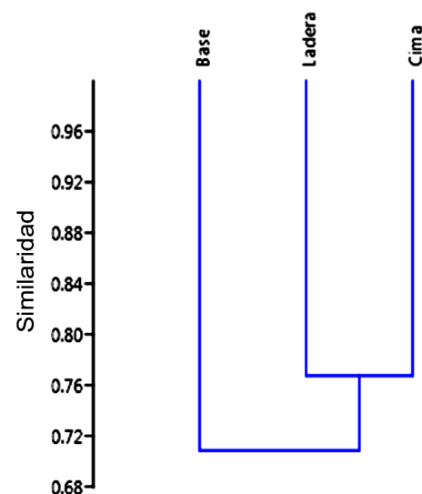
Figura 3. Dendrograma de Bray-Curtis, basado en los individuos arbóreos con un DAP \geq 10 cm revelados en las diferentes posiciones fisiográficas (cima, ladera, base), en el censo florístico realizado en la Unidad de Producción #6, El Dorado-Tumeremo, Bolívar-Venezuela.
