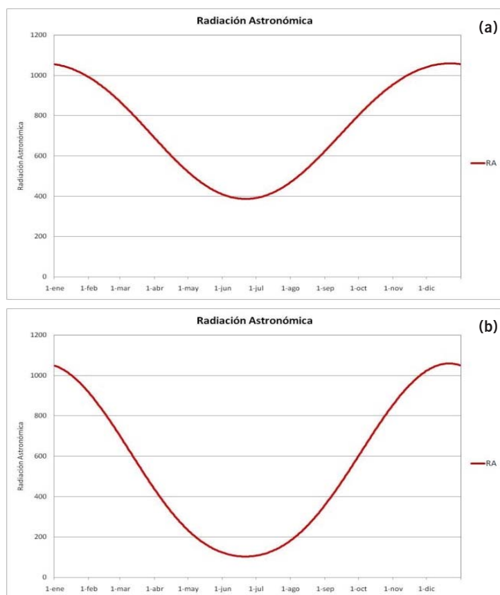
Figura 5. Radiación astronómica diaria (RA) en \text{cal/cm}^2\text{min} para Pergamino (a) y Ushuaia (b).
