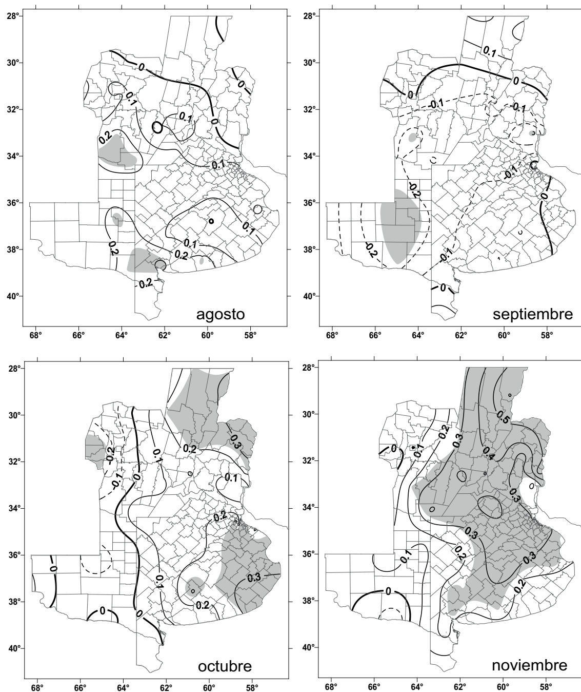
Figura 2. Correlación directa entre el índice BEST y la precipitación, de agosto a marzo, para el período 1950-2011. Sombra gris: área de correlaciones significativa al 10%.
